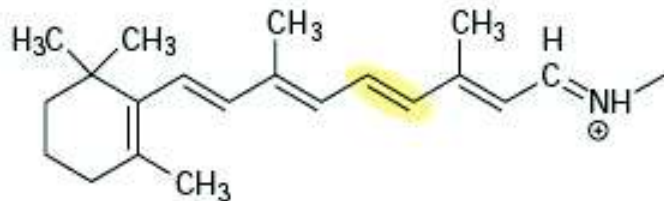
all-trans-Retinal
